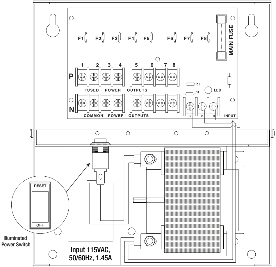
Fig. 2 - AL168175CB
