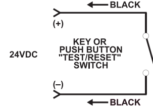
TEST/RESET
