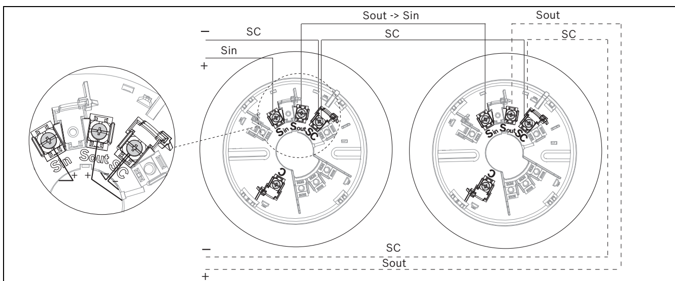
Figura 5.2 Fiação Classe B da Base com Isolador FAA-440-B6-ISO (Fiação Classe A Indicada pelo Cabo Tracejado)
