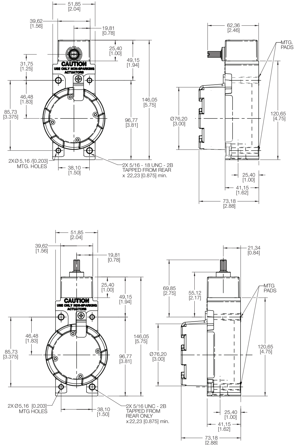
ABBILDUNG 12: EINBAUMASSE – nur als Richtwerte (mm/Zoll)
