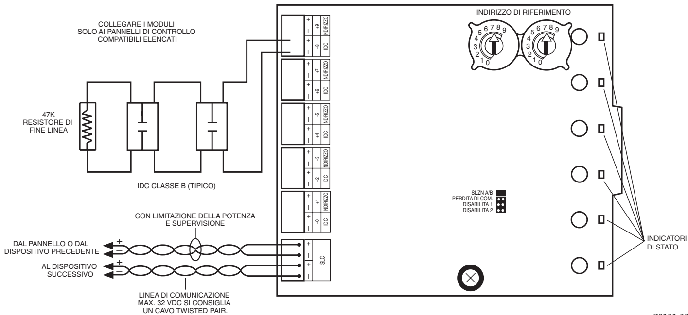
FIGURA 1: TIPICA CONFIGURAZIONE
