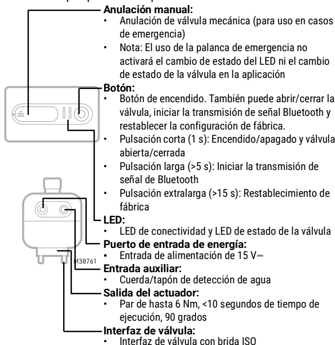
Fig. 2. Componentes
