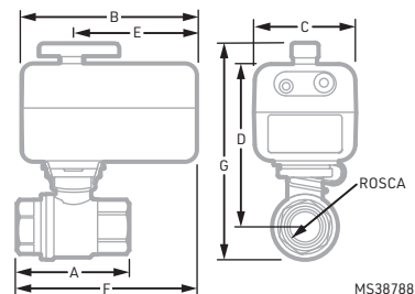
Fig. 7. Diagrama de dimensiones.
