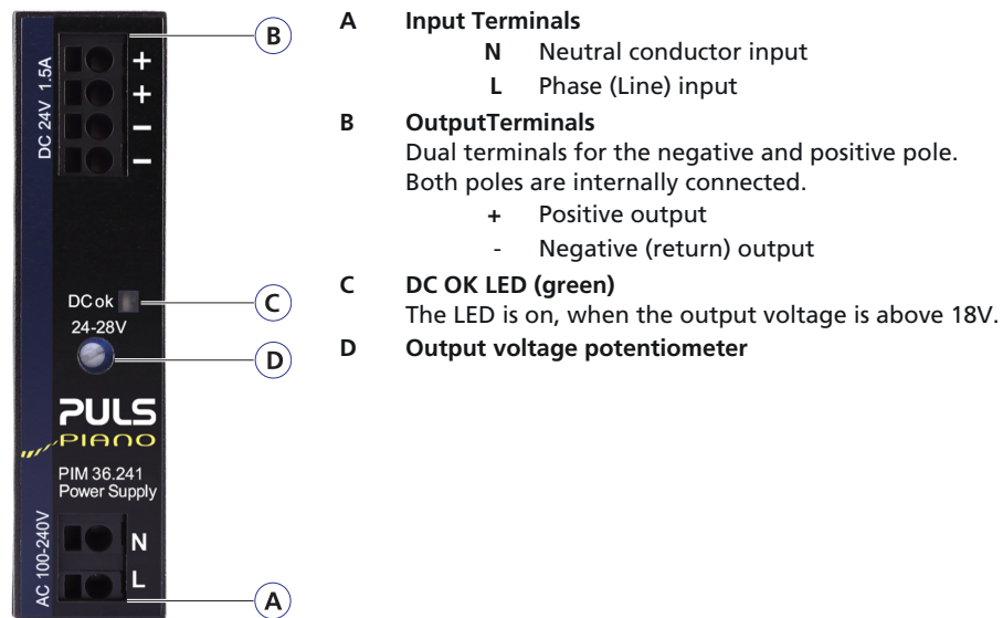
Fig. 13-1: Front side
