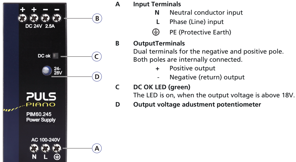
Fig. 13-1: Front side
