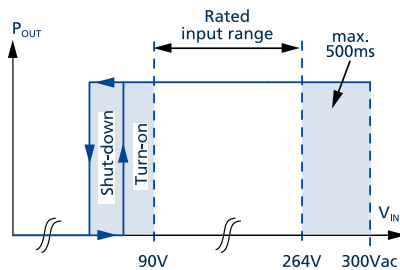
Fig. 3-1: Input voltage range
