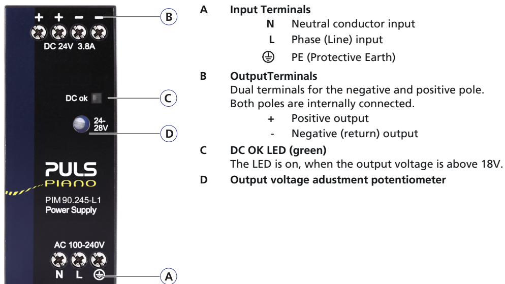
Fig. 13-1: Front side
