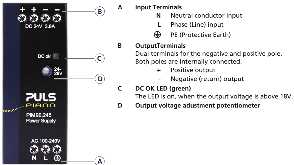
Fig. 13-1: Front side
