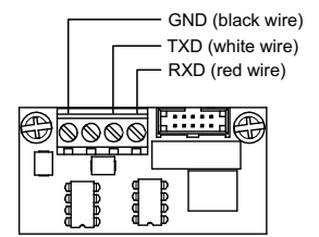
SA-232 wiring
